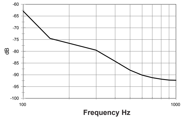
Типичное общее гармоническое искажение
