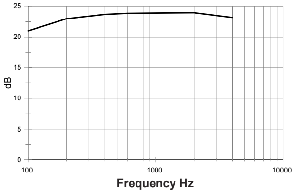
Типичное подавление отражения
