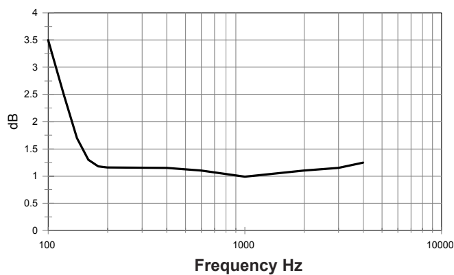
Типичное введенное затухание
